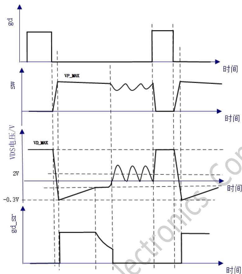
功能波形图
