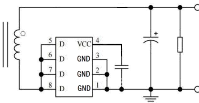
SR 放置在负端电路图
