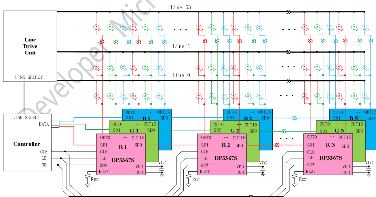
DP3367S 典型应用原理图
