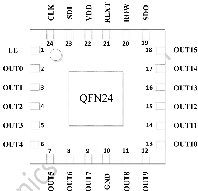
QFN24 引脚定义图
