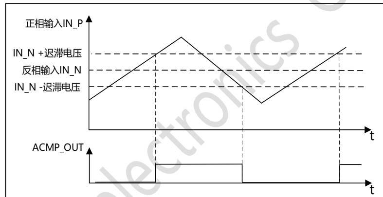
图 26-2 比较器迟滞
