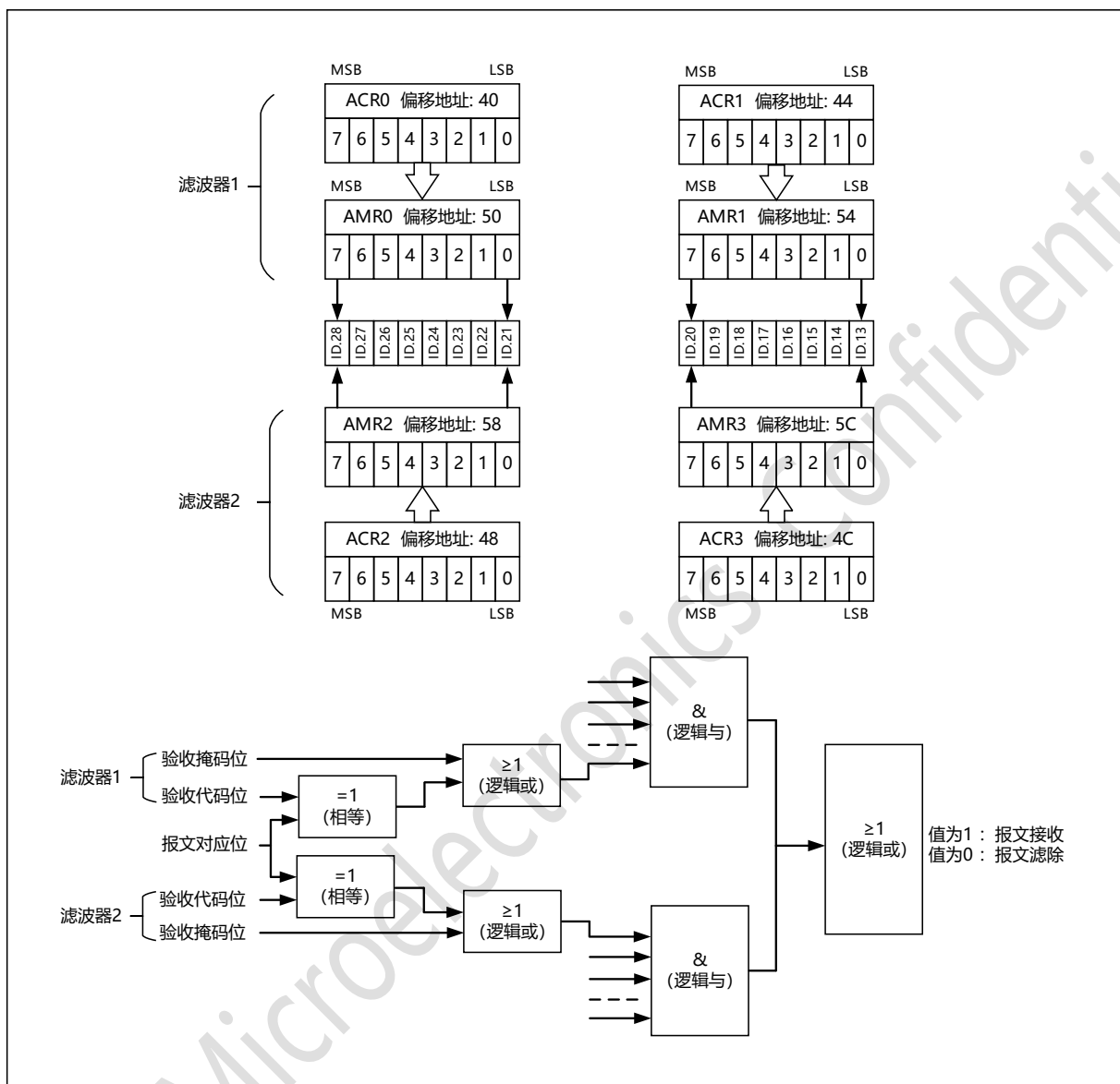
图 21-7 双滤波器模式接收扩展帧示意图
