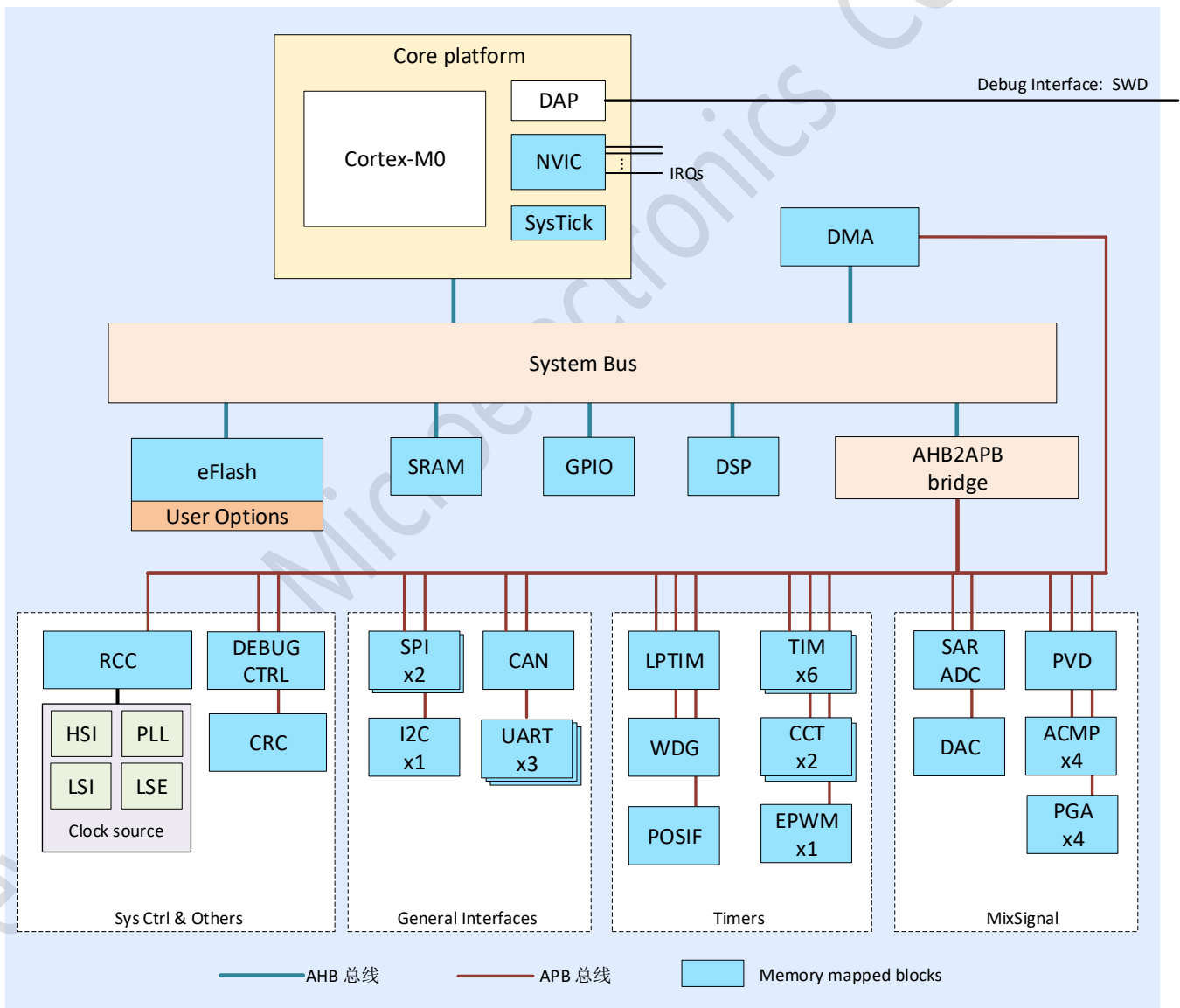
图 2-1 系统架构
