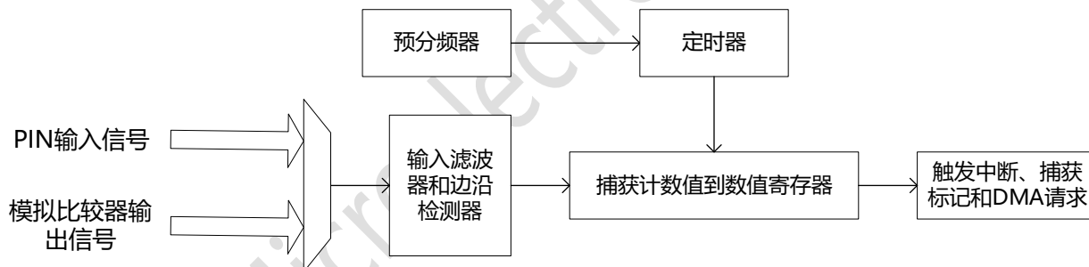
图 12-1 捕获模式
