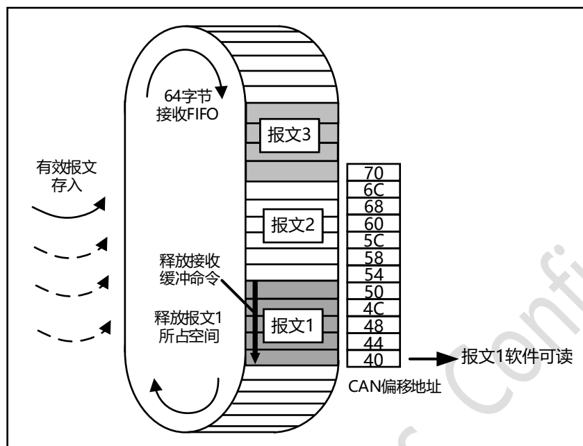
图 21-10 接收报文在接收缓冲的存储方式示意图
