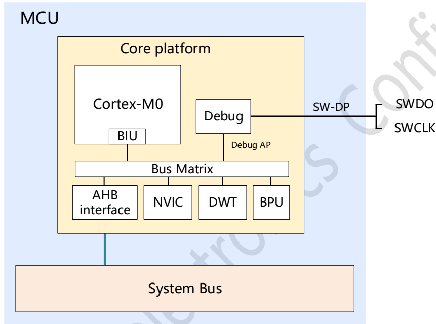
图 29-1 DPM32 MCU 和 Cortex®-M0 调试支持框图
