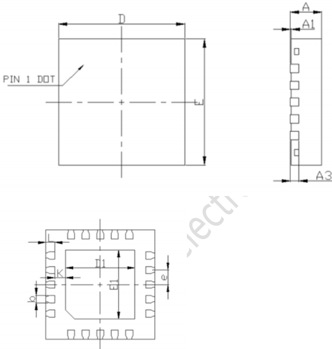
QFN3*3-20C-075 外观尺寸图
