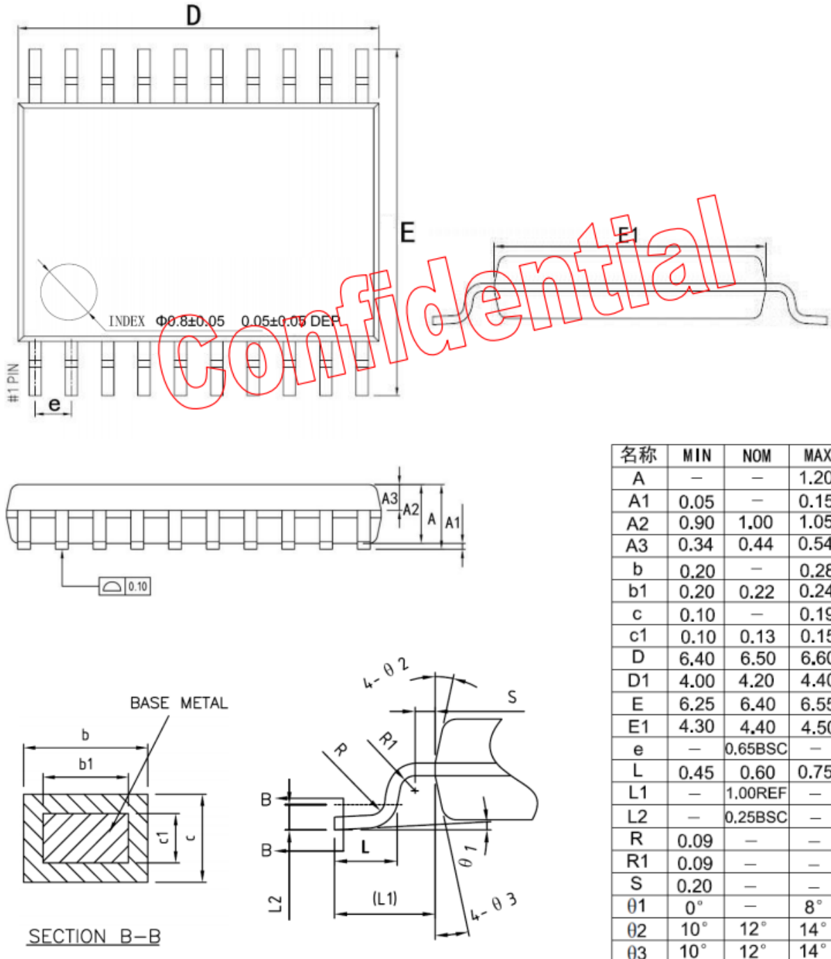
TSSOP20 外观尺寸图
